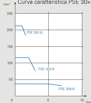
Curva caratteristica PSE 30x-8
